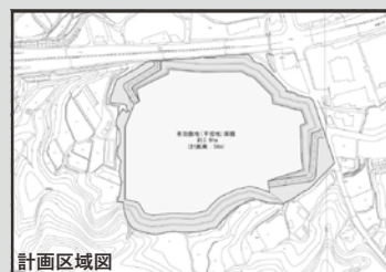
計画区域図
